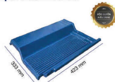
Ngói giả đá | Stone - like roof tile
